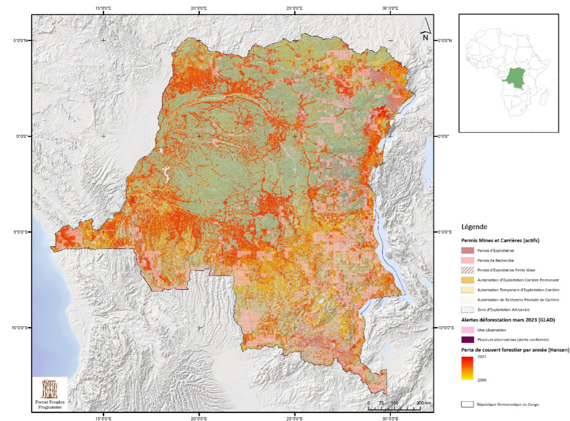
Figure 4 : Permis miniers et récentes alertes de déforestation GLAD.
