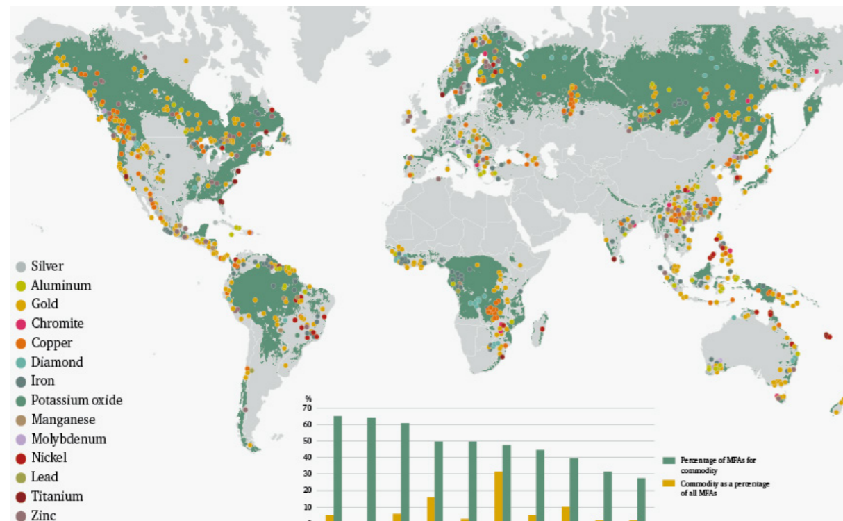
Figure 2 : Grandes exploitations minières dans les zones forestières par produit primaire.
